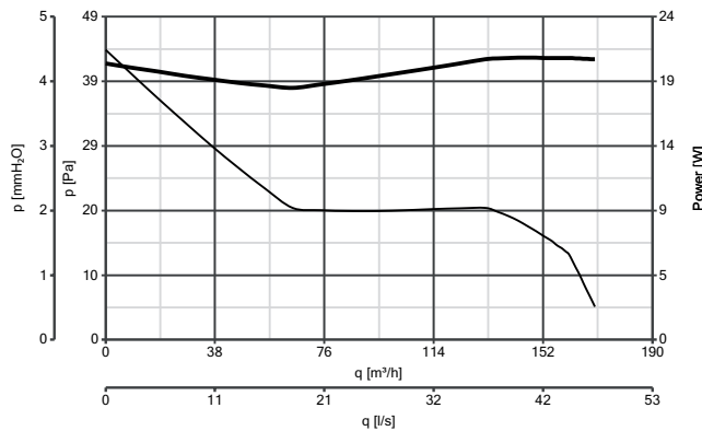
M 120/5" cod. 11301 - 11302 - 11311 - 11312 - 11321 - 11322 - 11331 - 11332 - 11692 - 11741 - 11746 - 11781 - 11782 - 11783 - 11784
