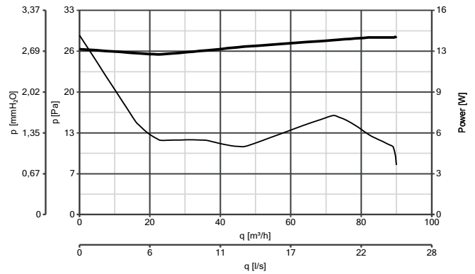
M 100/4" cod. 11201 - 11202 - 11203 - 11211 - 11212 - 11221 - 11222 - 11223 - 11231 - 11232 - 11614 - 11616 - 11646 - 11681 - 11682 - 11683 - 11684
