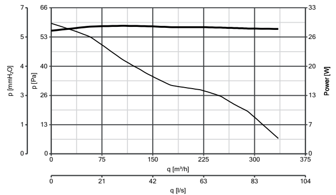
M 150/6" cod. 11401 - 11402 - 11411 - 11412 - 11421 - 11422 - 11431 - 11432 - 11698 - 11851 - 11856 - 11881 - 11882 - 11883 - 11884
